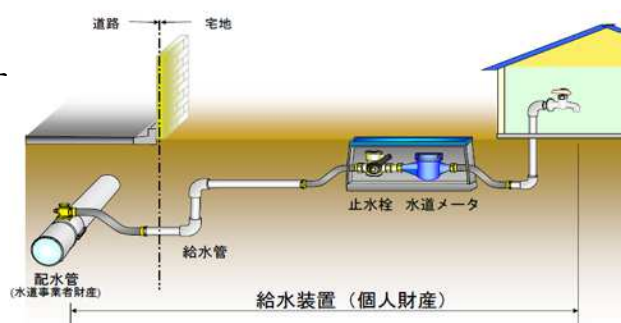
（参考）給水装置の概念図
